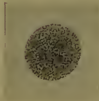
Fig. 221. Kolonien auf Gelatine 24 Stunden alt, mit Formol abgetötet. Vergr. 130fach (nach Weber).
